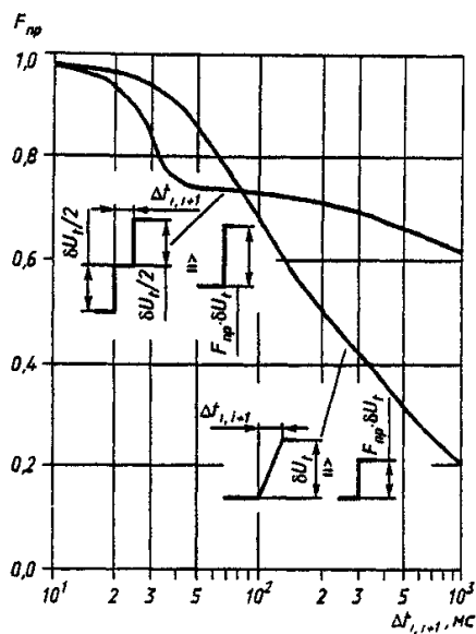
Рисунок В.1. Коэффициент приведения F_{np} для периодических колебаний напряжения, имеющих двухступенчатую и пилообразную форму
