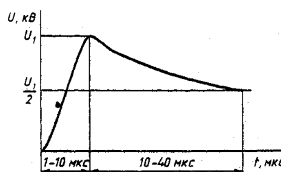
Рисунок Д.4. Форма грозových импульсов, характерная для точек присоединения б, e, ж на рисунке Д.1
