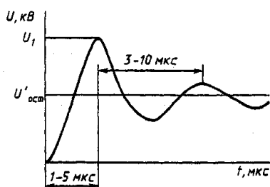
Рисунок Д.3. Форма грозových импульсов, характерная для точек присоединения, проходящих через выводы силового трансформатора, рассматриваемая обмотка которого имеет связь с ВЛ (точки присоединения з, з', u на рисунке Д.1)
